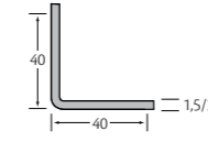
40 x 40 x 1 mm (RVS) gelijkzijdig hoekprofiel 1x3m. Art.nr.: 518
