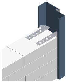
inmetselkozijn
