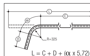
Binnenhoek (vaste straal)
