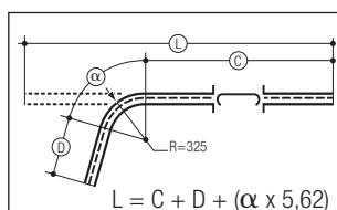
Buitenhoek (vaste straal)
