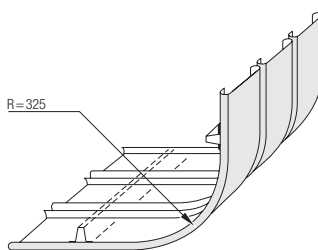
Buitenhoek (vaste straal)
