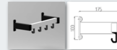
Wandgarderobe VK 2
