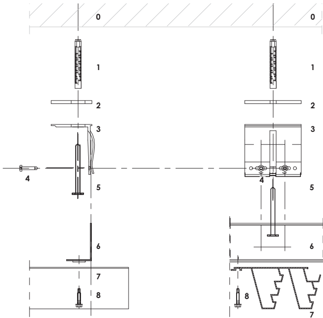
Horizontale doorsnede
