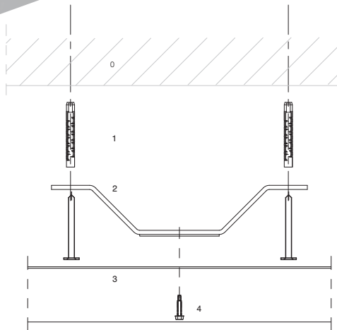
Horizontale doorsnede
