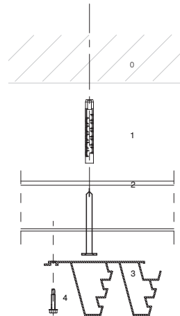
Verticale doorsnede
