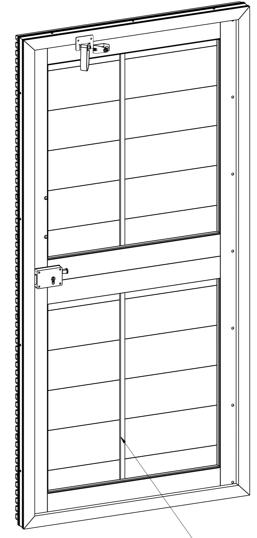
SCALE 1:10 3D Achteraanzicht verstivingsprofiel bij kozijn > 892mm
