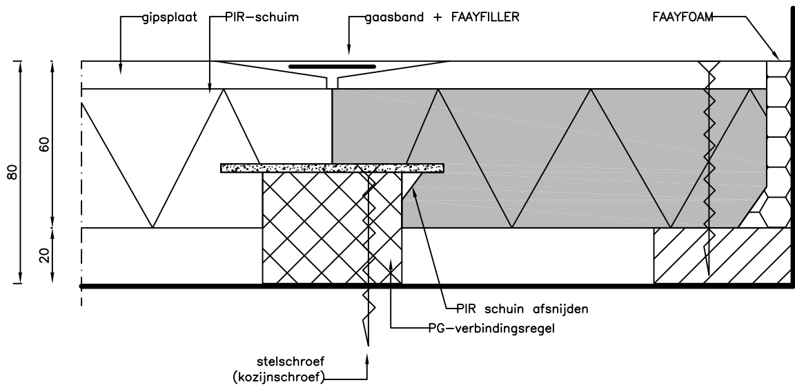
koppeling sluitpaneel PG-wand
