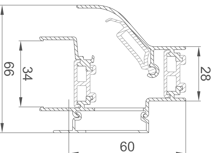
Smart 60 / 34
