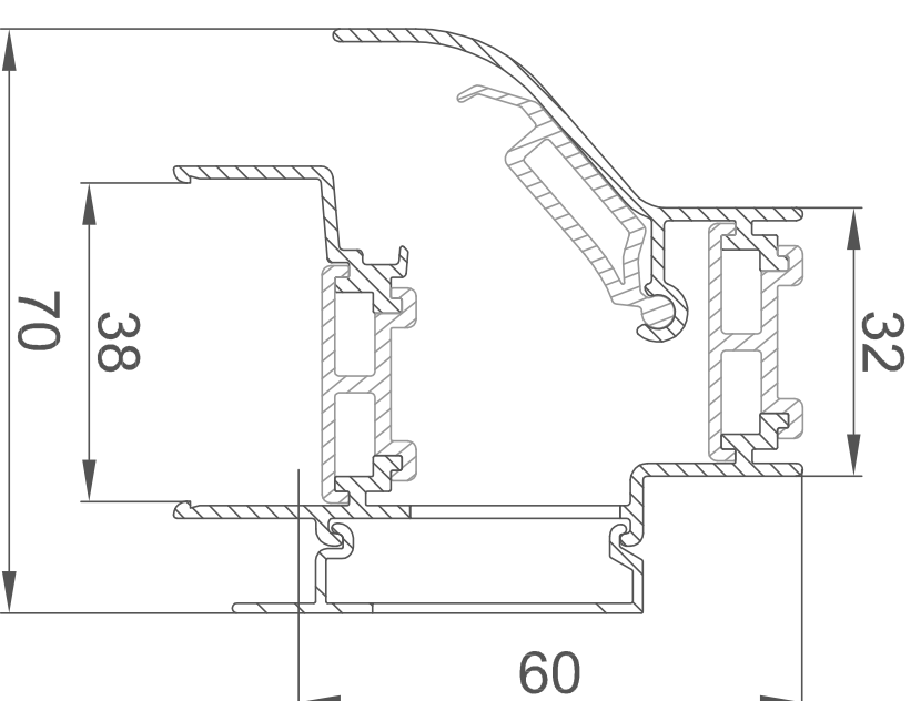
Smart 60 / 38
