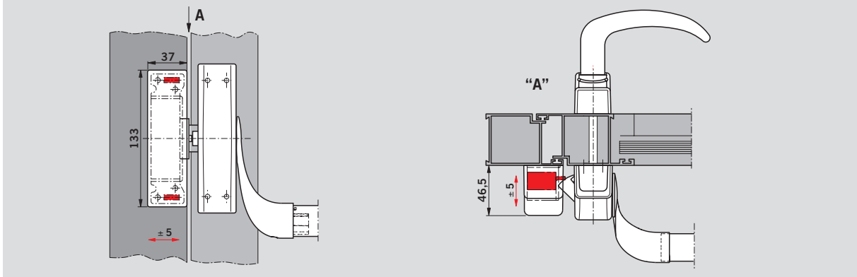
Toepassingsvoorbeeld PHX 50 met PHA 2000 in Contur design op een profieldeur
