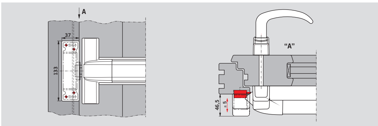
Toepassingsvoorbeeld PHX 50 met PHB 2000 in Contur design op een profieldeur
