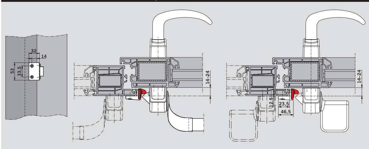
Toepassingsvoorbeeld PHX 22 op een deur met aanslagprofiel, universeel toepasbaar op 1- en 2-vleugelige deuren
