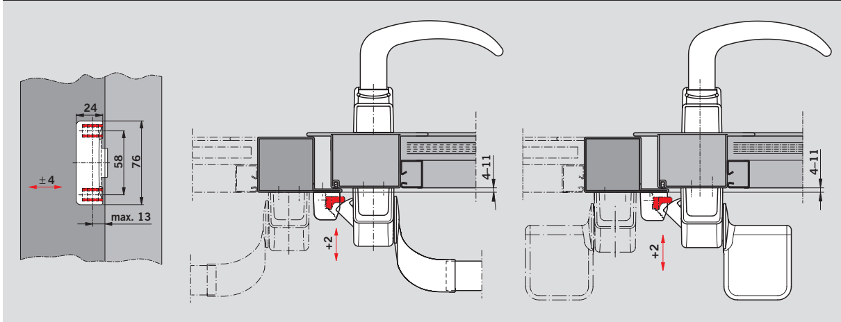
Toepassingsvoorbeeld PHX 21 op een opdeksleur, universeel toepasbaar op 1- en 2-vleugelige deuren
