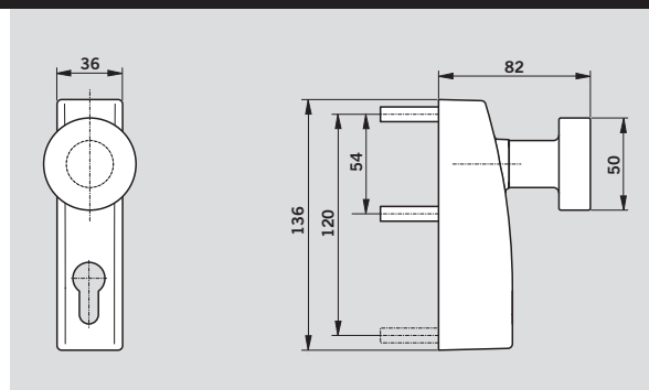
PHT 06 – buitenbeslag met knopkruk
