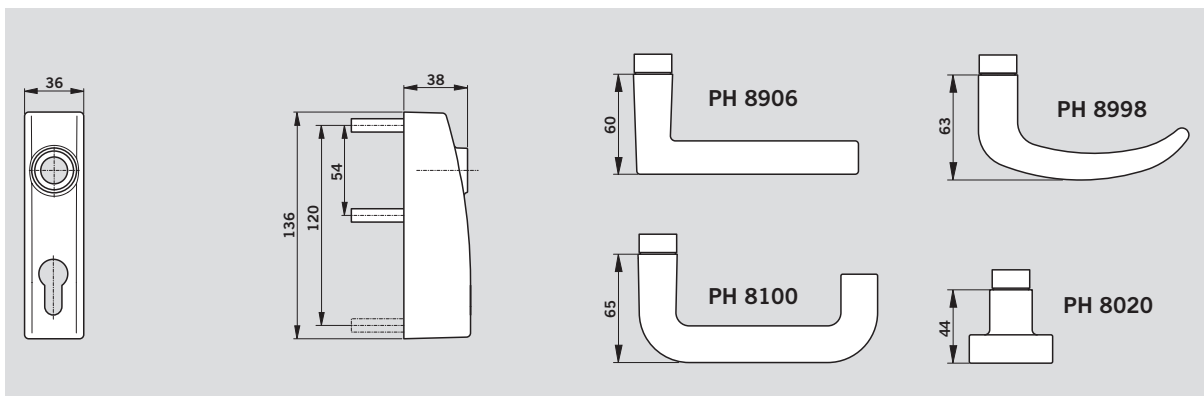
PHT 07 – buitenbeslag modulair
