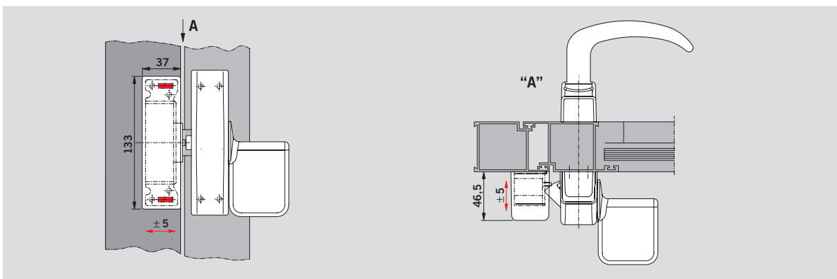
Toepassingsvoorbeeld PHX 50 met Exit Pad in Contur design op een profieldeur
