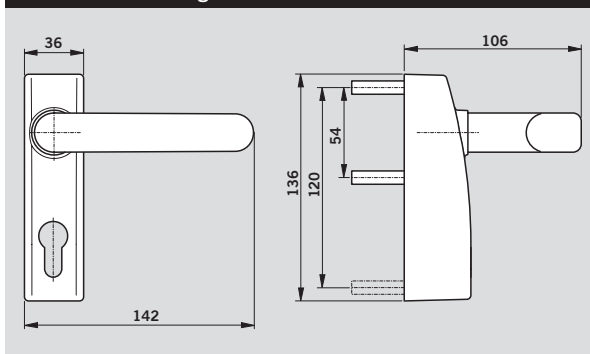
PHT 01, 03, 05 – buitenbeslag met deurkruk
