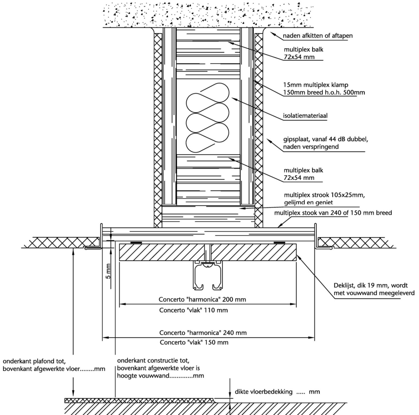
Tekening BVD1
