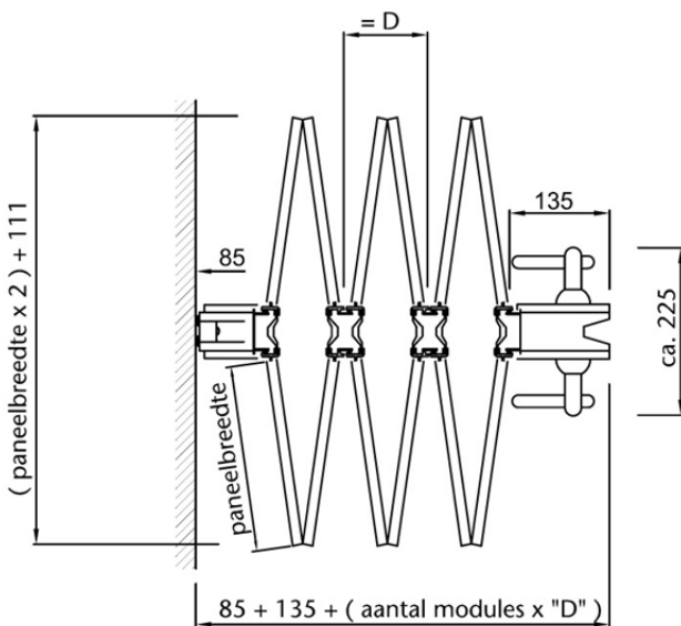
Tekening VD3
