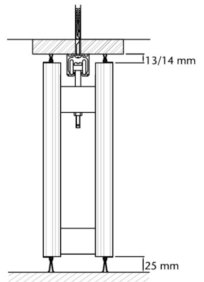
Tekening VD4
