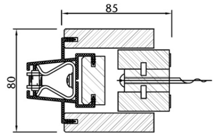
Tekening VD2
