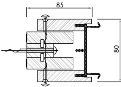
Tekening VD1
