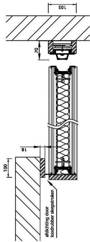
Detail zij / muuraansluiting
