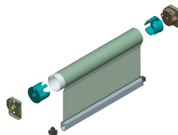
Zonweringdoek (Standaard handbediening) Motorische uitvoering mogelijk
