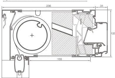
→ DucoTwin 120 'ZR' AK Alto
