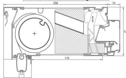
→ TronicTwin 120 Largo (AK)
