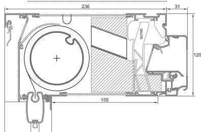
→ TronicTwin 120 Alto (AK)
