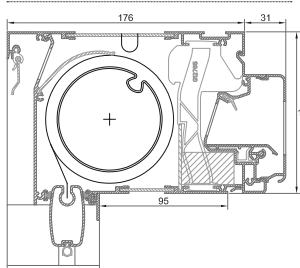
→ DucoTwin 120 'ZR' Corto
