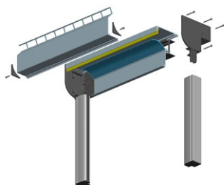
Zonweringkast DucoTwin 50 'ZR'
