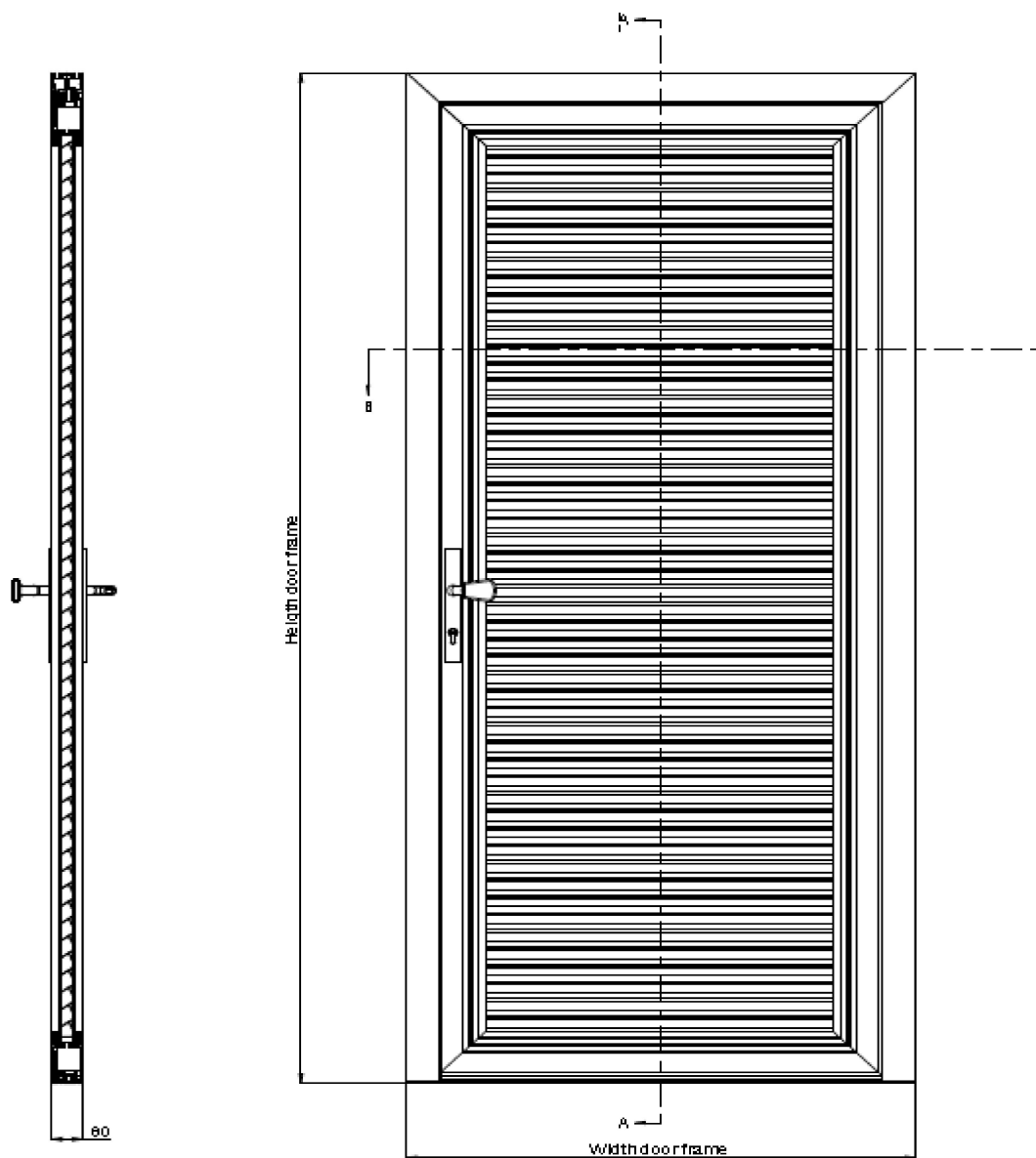
Section A-A
