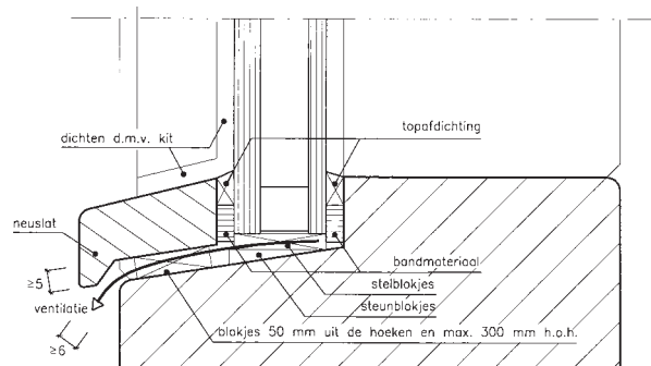
Neuslatten voor een goede vochtafvoer.
