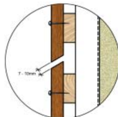
Voorkom capillaire naden.
