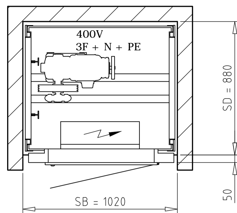
MACHINEKAMER GEINTEGREERD IN BOVENZIJDIGE SCHACHT
